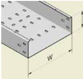
Khay Cáp - Cable Tray
